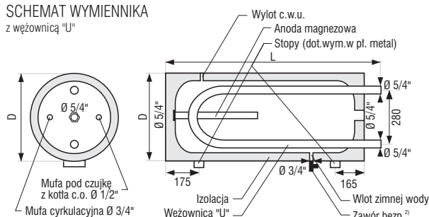
SCHEMAT WYMIENNIKA z podwójną węzownicą "U"
