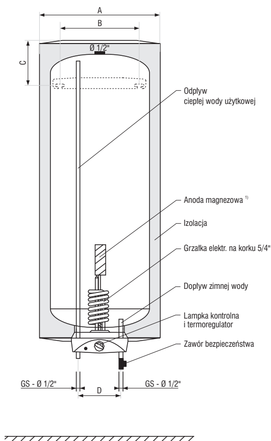
SCHEMAT OGRZEWACZA poj. 30-80 l.
